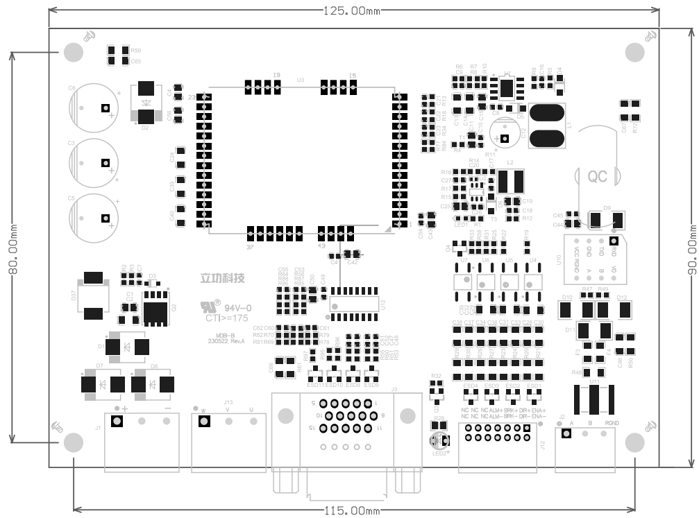
图 7.1 MDB20x-A 板尺寸图
