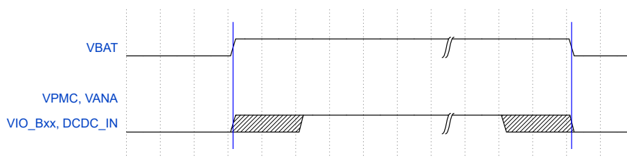
图 4: 上电时序要求
