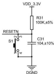
图 1.8 复位电路
