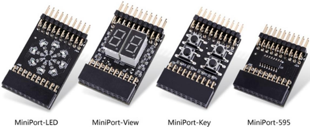
图 1.26 MiniPort 模块
