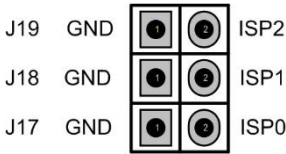
图 1.16 ISP 接口引脚
