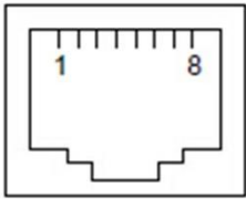
图 1.22 RJ45 引脚排列
