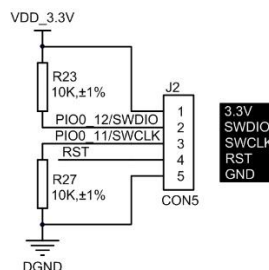
图 1.9 调试电路
