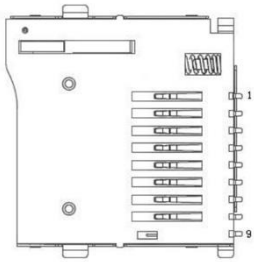
图 1.25 TF 卡接口
