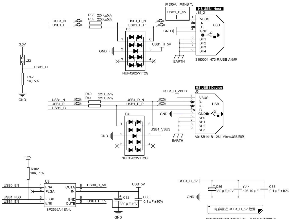
图 1.6 USB1 电路
