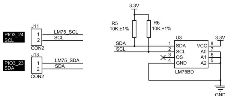
图 1.13 LM75B 电路
