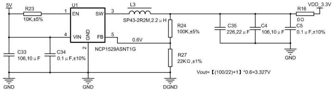
图 1.3 NCP1529 电源电路
