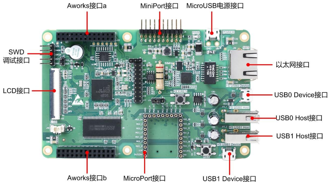
图 1.2 Easy-54608M4 开发板正面图片
