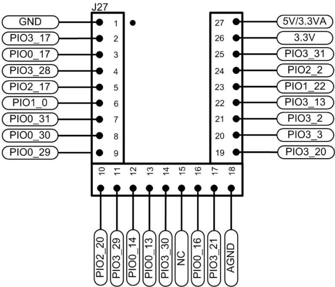
图 1.18 Easy-54608M4 MicroPort 引脚分配示意图
