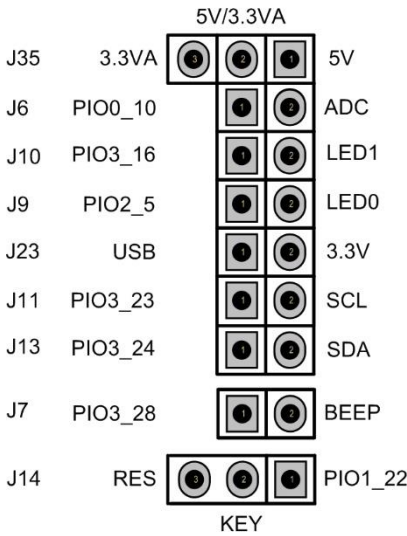
图 1.15 板载外设接口引脚图示
