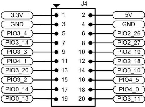
图 1.17 Easy-54608M4 MiniPort 接口图示
