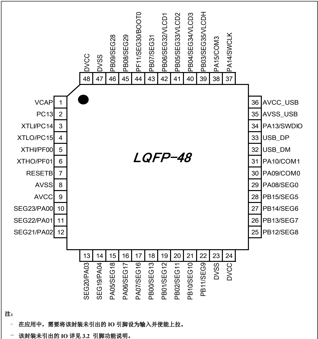
图 3-1 封装示意图
