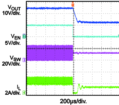
EN Shutdown I_{OUT}=1A
