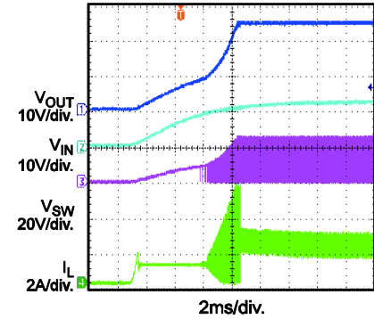
VIN Startup I_{OUT}=1A
