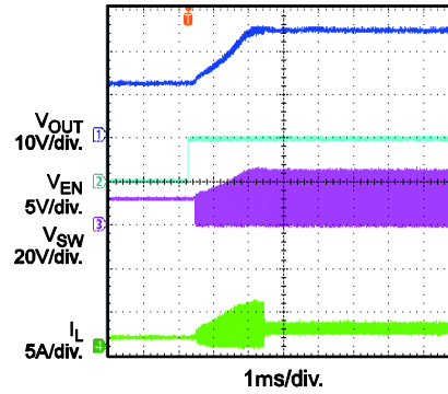
EN Startup I_{OUT}=1A
