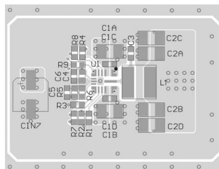
Top Layer
