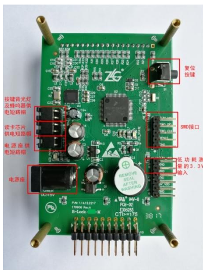
图 1 实物背面图
